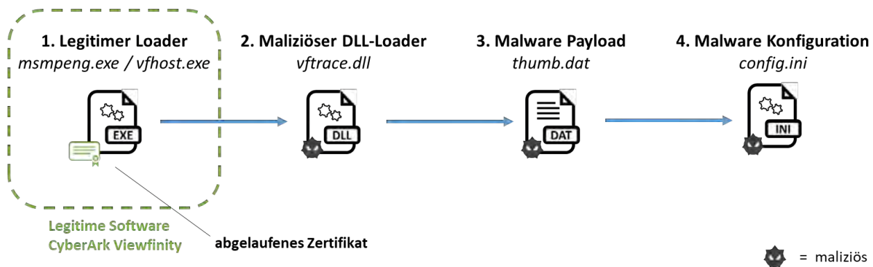
Abbildung 1: Komponenten von HYPERBRO
